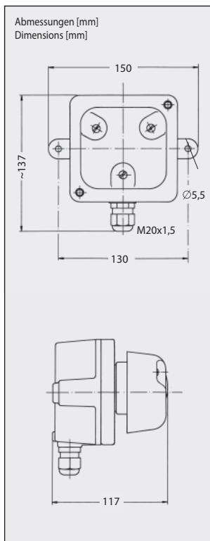
Abmessungen Physical dimensions
