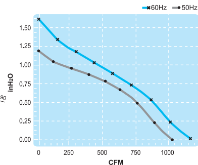
(Centrifugal Fan)
