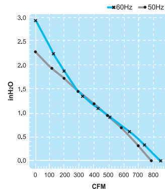
(Centrifugal Fan)
