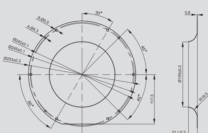
220A (For UF220APA)
